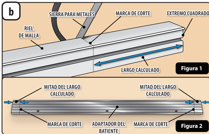
Riel de malla (C/D)
