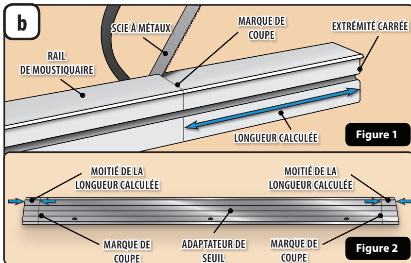
Rails de moustiquaire (C/D)
