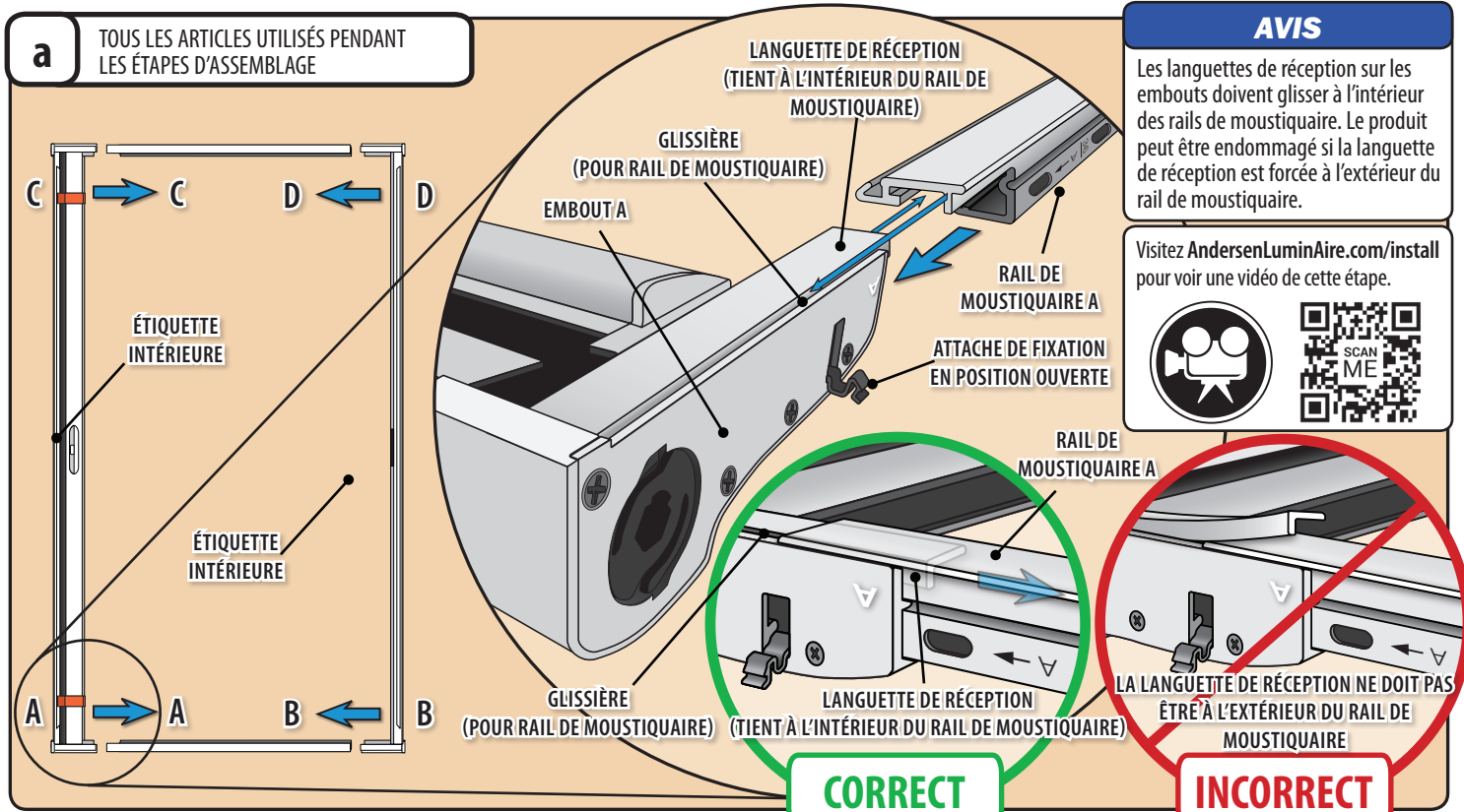
Rails de moustiquaire (A/B)
